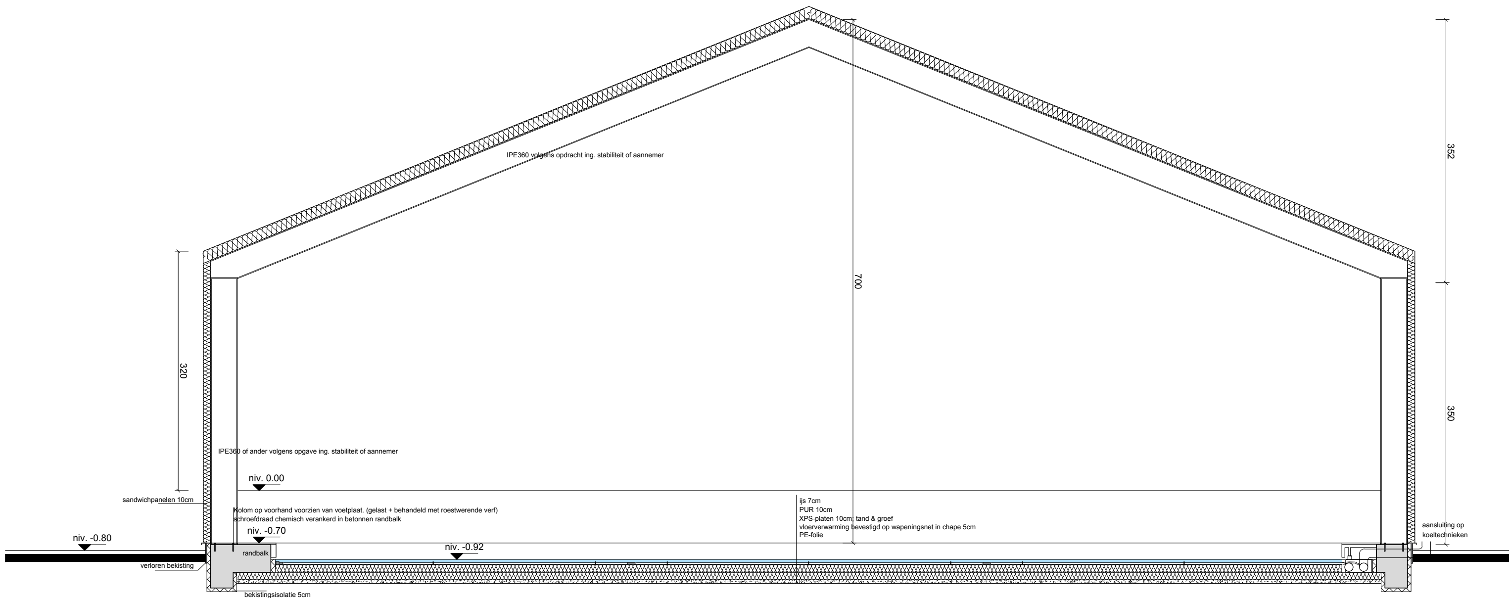
Snede A schaal 1/50
